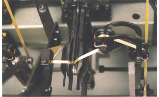
Band auf Wickeldorn geklemmt
